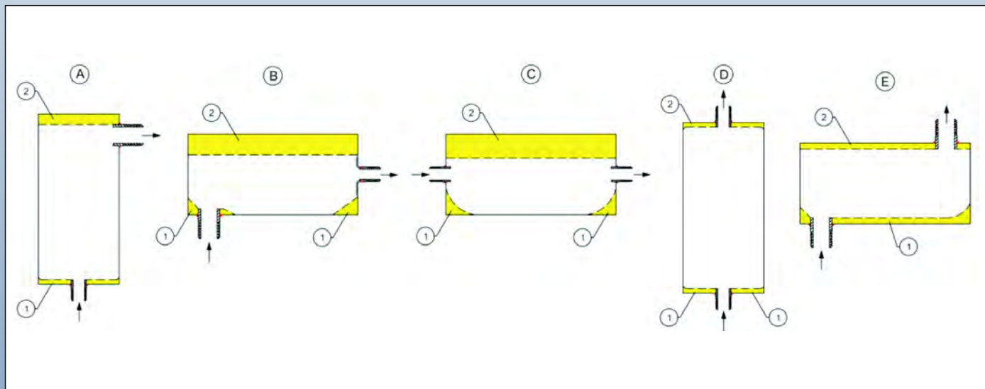
图片A, B, C, D, E展示出错误的想法及热水器不良的安装位置，带有 污物沉积的地方 (1)或 空气积聚 (2)以及还有内部尖角有助于颗粒的积聚。
