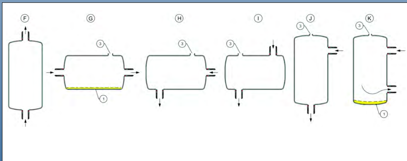
图纸F, H, I, J展示了带有圆角的设计。通过位置(F)，或气孔(3)的存在避免了空气凹位。如果按照流向流动的，可避免污物沉积。附图G和K展示了污物沉积的危险，并可能在最低部(1)要求要有一个排放孔。
