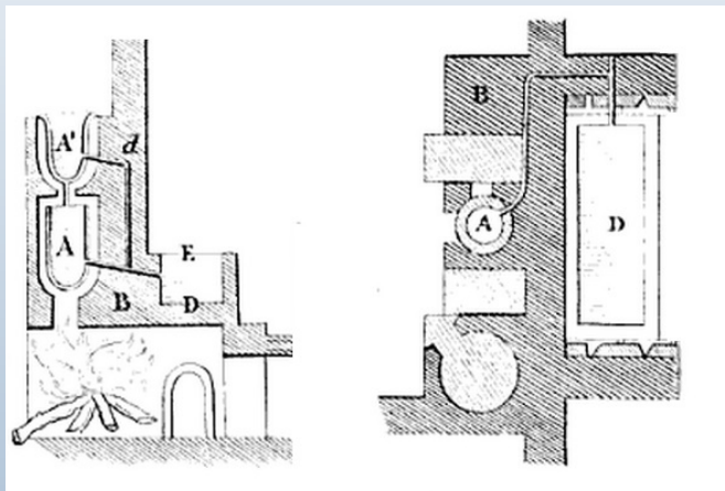
上图：在庞培的一座罗马别墅里热水浴的部分，使用热虹吸的原理，带有两个蓄水池A，并且A通过管D将水供应至澡盆D。 (Voyage pittoresque ou Description des royaumes de Naples et de Sicile, par l'abbé de Saint-Non (1781), vol 2).
