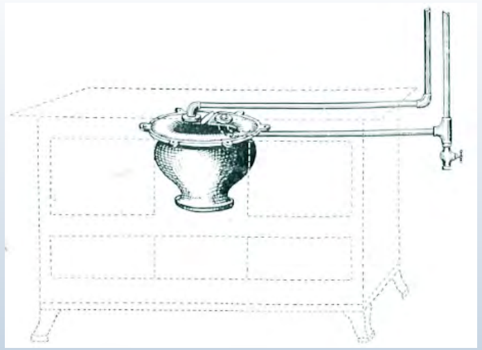
换热器锅炉安装在炉子里面 (Ets Demoulin目录书, Farciennes, 1932, Ultimheat博物馆)
