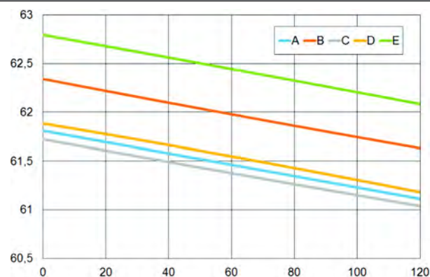
在0.25°C/分低温下降基础上的反应时间
