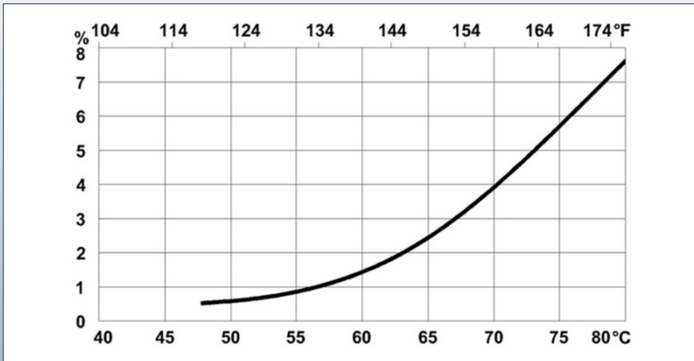
K-2 水垢沉淀与温度的对比
