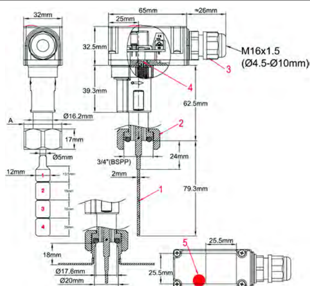
1: 浆叶 2: 塑料主体和塑料的 3/4" BSPP接头螺母 3: PA66电缆接头 4: 微型设定值调节刻度盘 5: 指示灯
