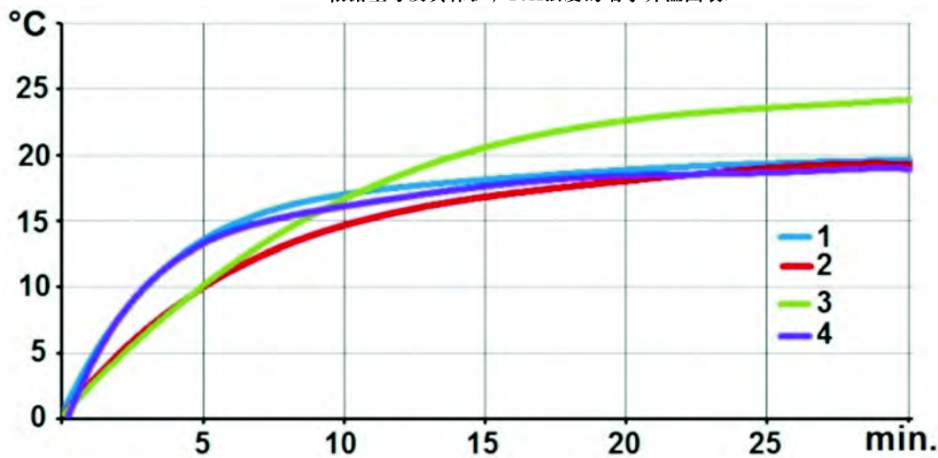
根据型号及其保护，16A强度的端子升温图表。
