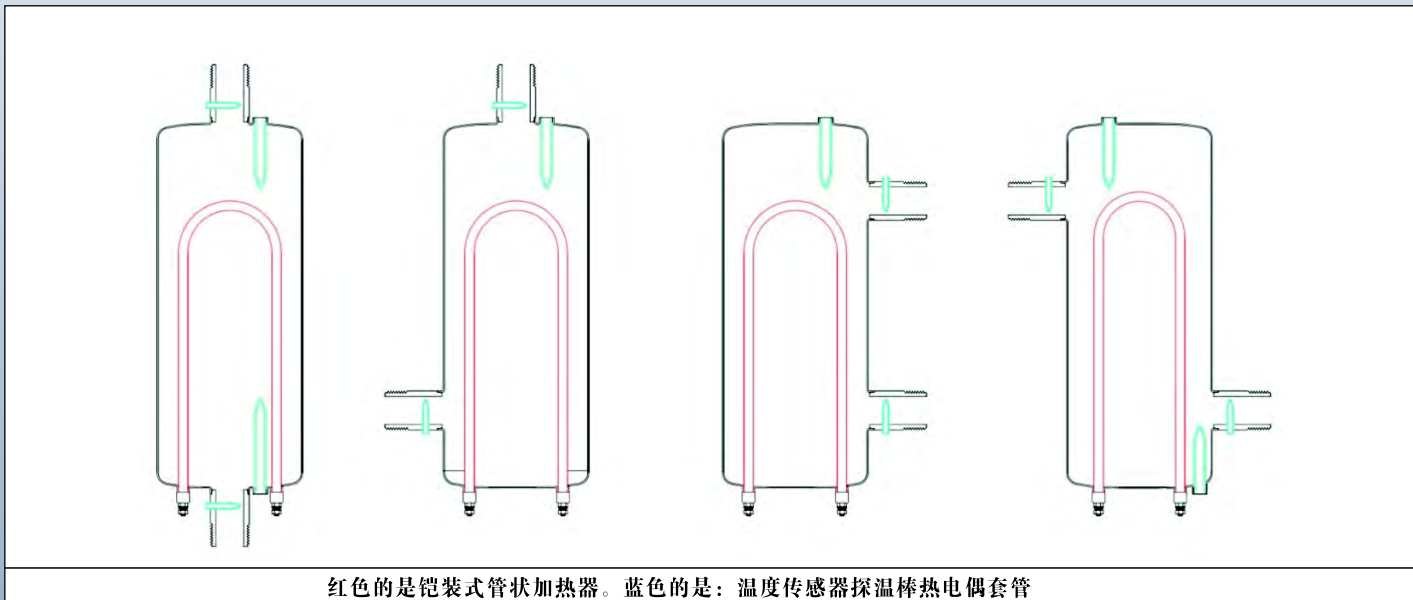
用于温度传感器热电偶套管的首选位置
